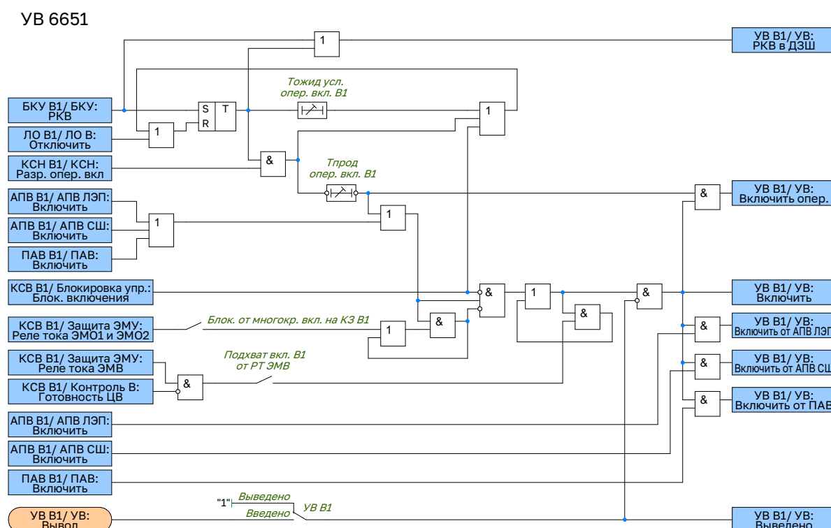
Рисунок 2.80 – Функциональная схема управления выключателем В1
