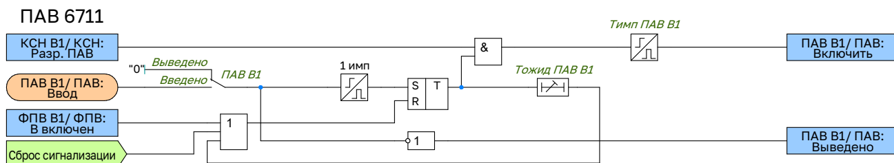
Рисунок 2.71 – Функциональная схема логики ПАВ В1
